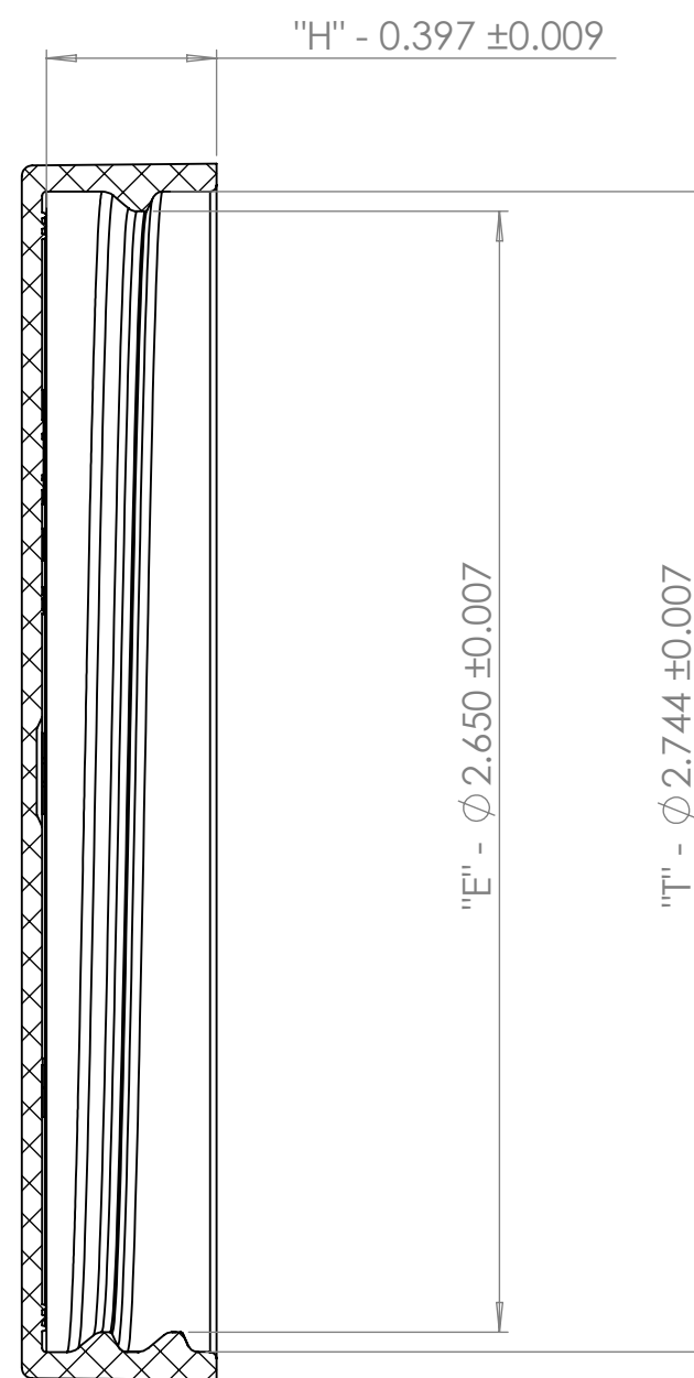
SECTION A-A
